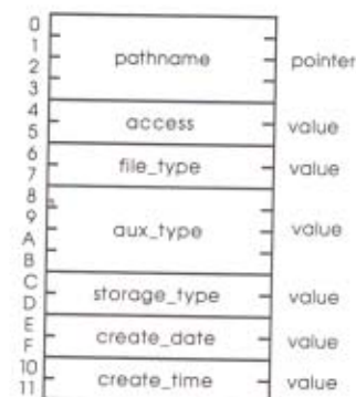
CREATE ($01) Parameter block
