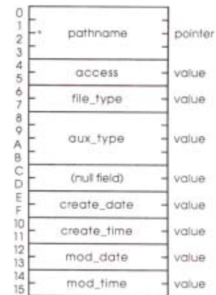
SET_FILE_INFO ($05) Parameter block
