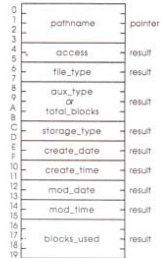
GET_FILE_INFO ($06) Parameter block
