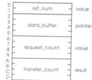
READ ($12) Parameter block
